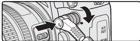
Подключение GP1-CA10 кабеля к D3 цифровой фотокамере
