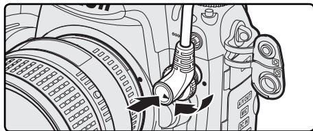
Podłączanie GP1-CA10A do cyfrowego aparatu D3S
