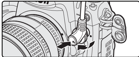
Tilslutning af GP1-CA10A til et D3S digitalkamera
