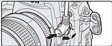
Collegamento di GP1-CA10A a una fotocamera digitale D3S
