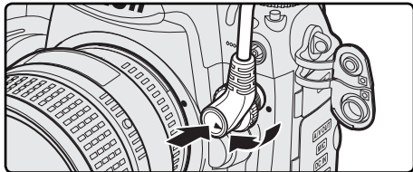
GP1-CA10A:n kytkeminen D3S-digitaalikameraan
